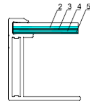
Section A-A 6:1
