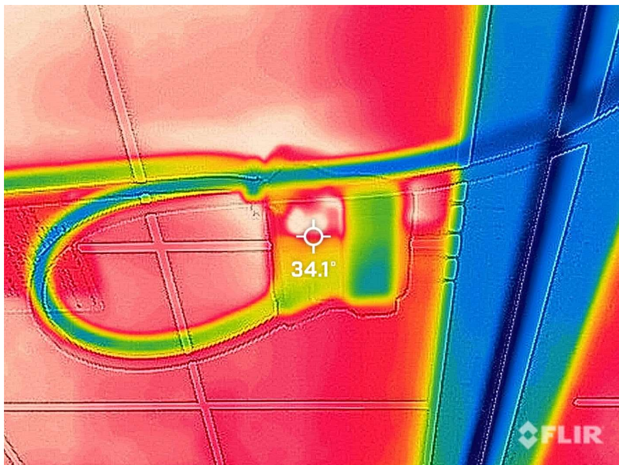
リマテック太陽光発電所(岡山) クラスタ落ちパネル測定写真(2023年3月~4月)
