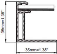
Section A-A 8:1
