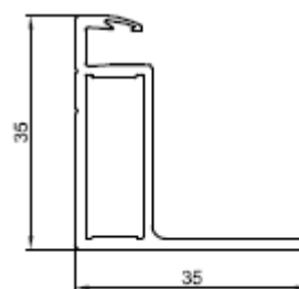
Section A-A 10:1
